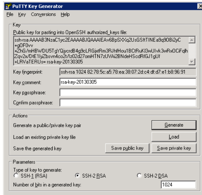
図 7: PuTTYgen*
